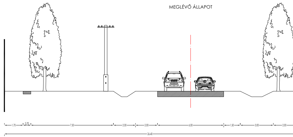
③ GÁT U. MEGLÉVŐ ÁLLAPOT
