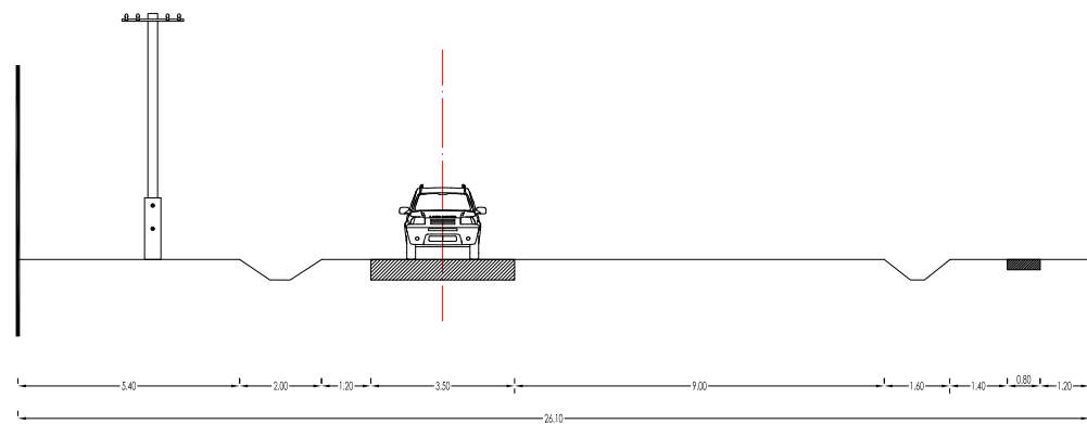
④ RÁKÓCZI U. MEGLÉVŐ ÁLLAPOT
