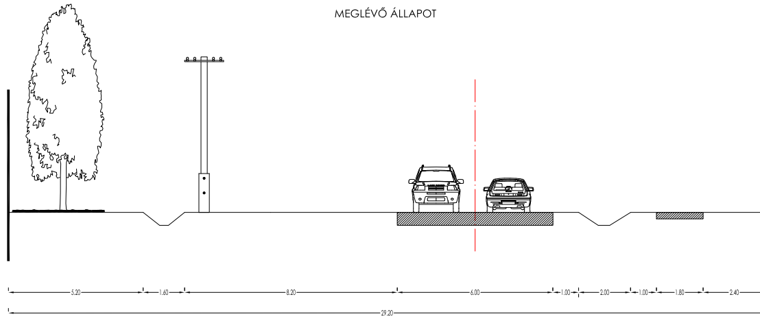
② PETŐFI U. MEGLÉVŐ ÁLLAPOT
